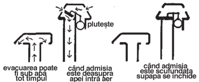
ILUSTRARE SIMPLĂ A PRINCIPIULUI SNORKEL
